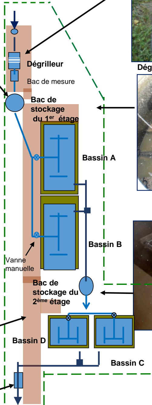
2 ème étage : bac de stockage, bassins C et D
